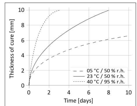
Diagram 1: Hitrost utrjevanja Sikasil® WS-305 EU
